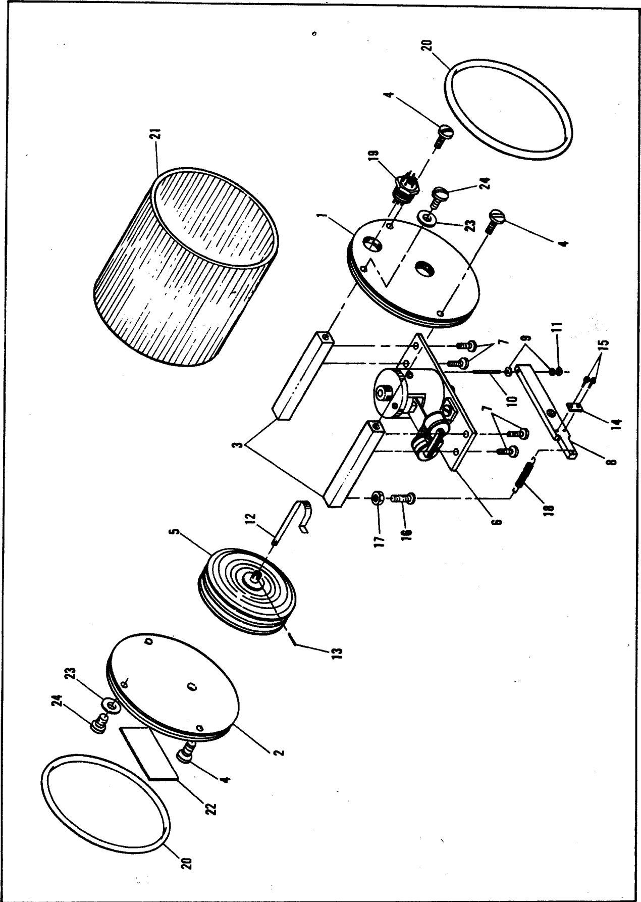
1C407 Altitude Hold
